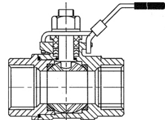
Robinet tournant sphérique Ball Valve Kugelhahn
